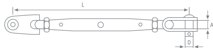
Tenditori snodati a due forcelle Two toggles
