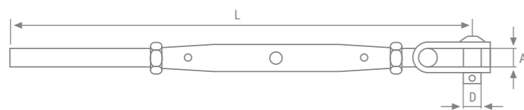
Tenditori snodati con terminale a pressare Toggle and swaging terminal
